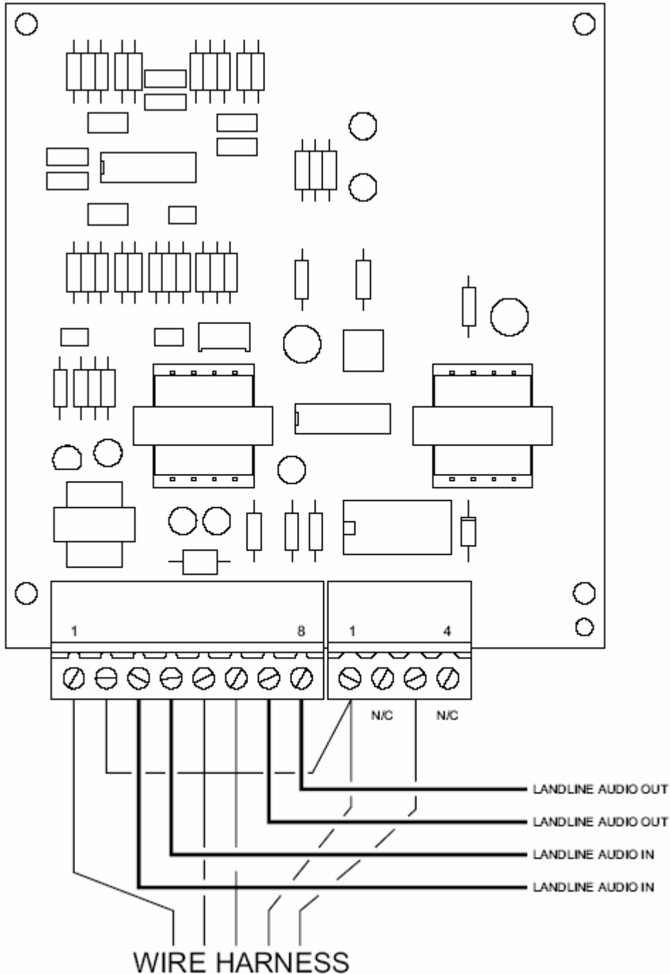
Fig. 13: Landline Wiring
